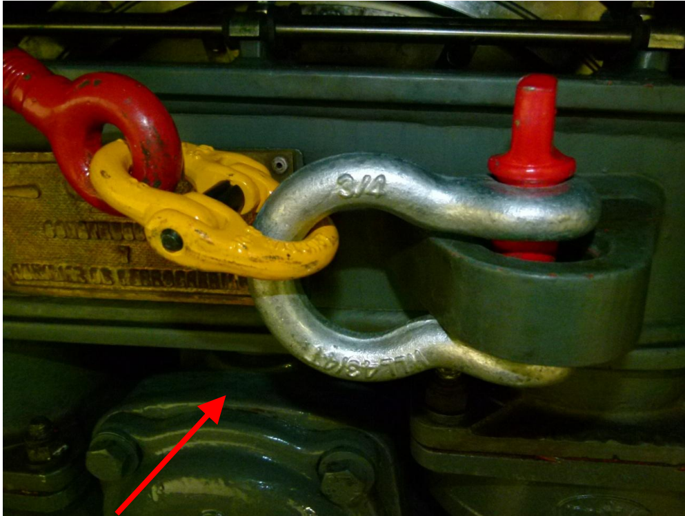
Imagen 1 – Fijación del cáncamo a la oreja de izaje del bogie con grillete lira con bulón roscado de 4,75 Tn
