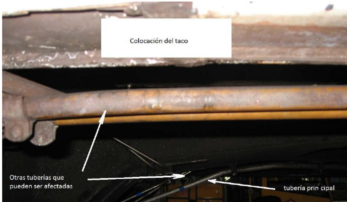
Imagen 7 – Vista de las cañerías a sortear en el izaje.
