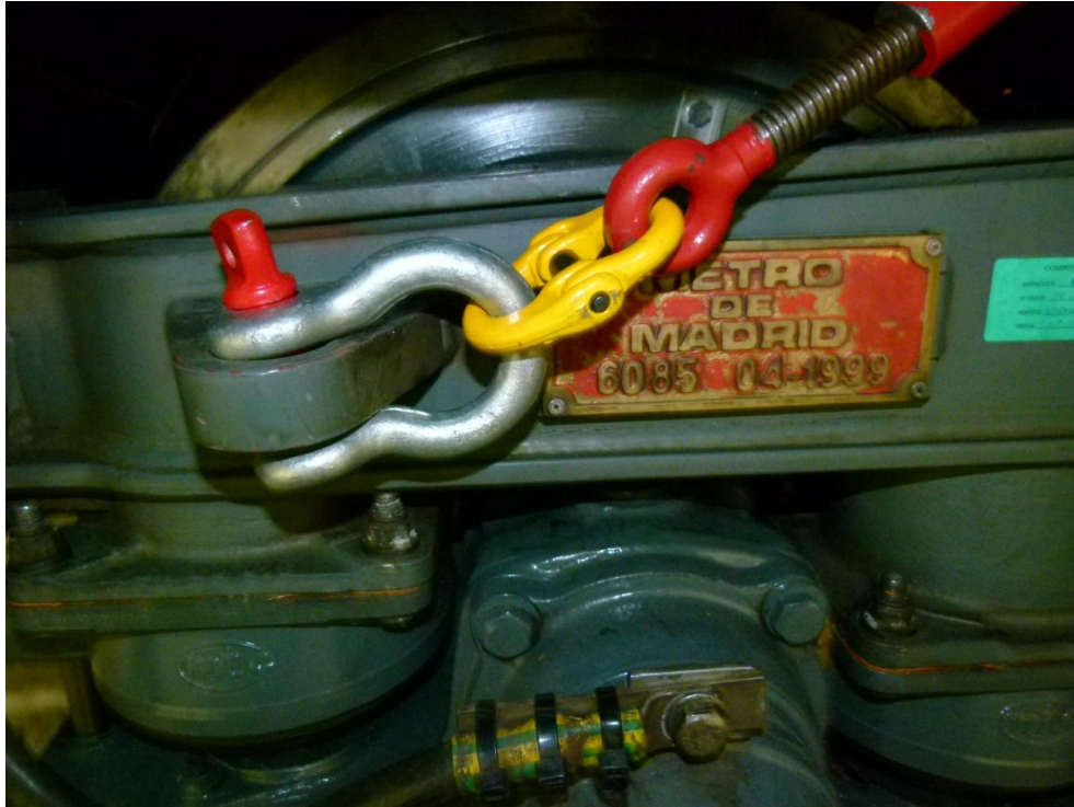
Imagen 5 – Fijación en el bogie
