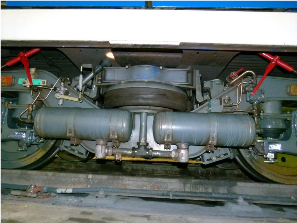
Imagen 3 – Vista frontal de bogie, posición de anclaje de los bogies a los travesaños del bastidor
