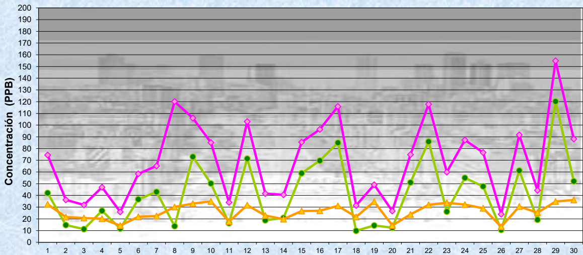
ABRIL 2026 Concentración promedios de 8 hs de 16 a 24 Hs
