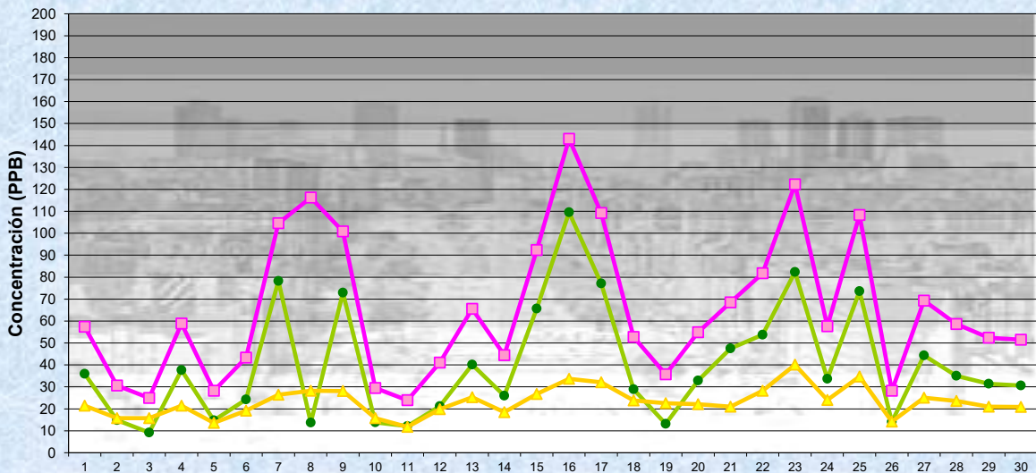
ABRIL 2026 Concentración promedios de 8 hs de 8 a 16 Hs
