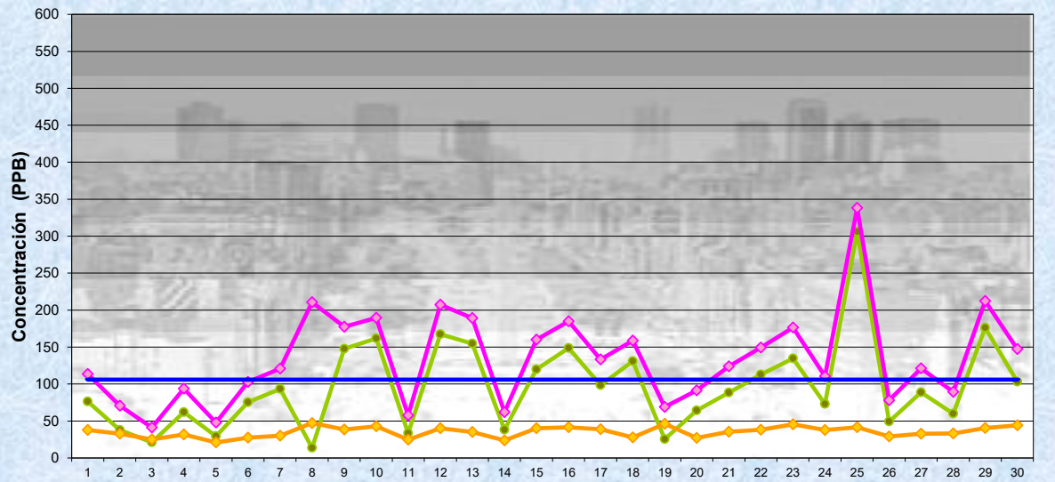
ABRIL 2026 Concentración Máxima de promedios de 1 hora
