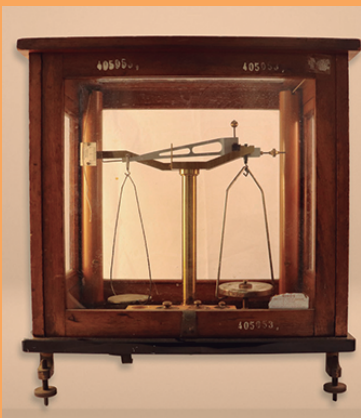
BALANZA DE PRECISIÓN A PÉNDULO 1913
