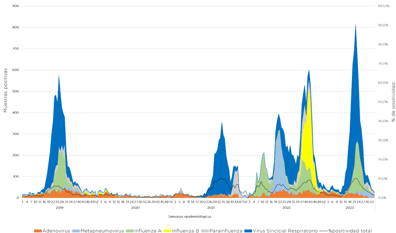
Gráfico 1. Muestras positivas según virus y porcentaje de positividad. Año 2019 n= 6744; Año 2020 n= 654; Año 2021 n=4122; Año 2022 n= 11404, Año 2023 (h SE 33) n=6773
